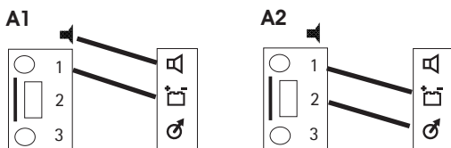
Installeringsalternativer med monolyd.
