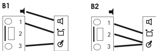
Installeringsalternativer med stereolyd.
